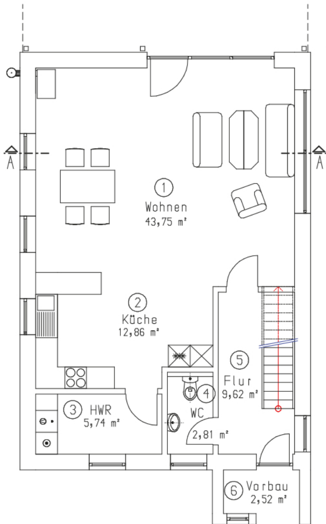
Erdgeschoß
